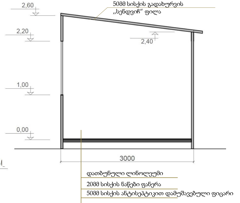
ჭრილი 1-1.
